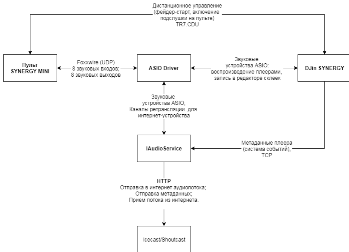
Схема взаимодействия приложений с пультом
