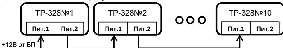
Рисунок 2.10 – Питание нескольких TP-328 от одного БП
