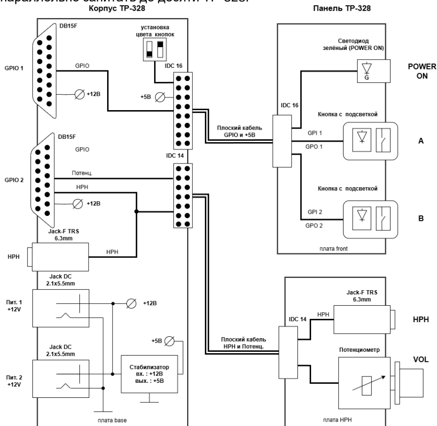
Рисунок 2.5 - TP-328. Схема структурная
