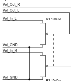
Рисунок 2.7 – Схема регулировки громкости наушников
