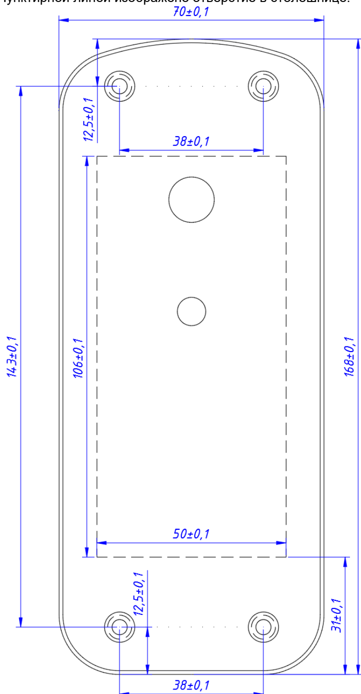
Рисунок 3.1 – TP-328, шаблон для монтажа
